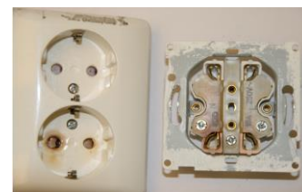
Fig 8 – Skade / varmgang kontakt ved manglende avlastning
